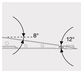
MFL 112 Bakparti med fällbar påkörningsläpp med rullbart gångjärn. Passar ej på släp.
