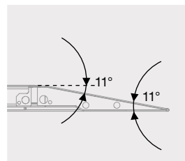
MFL 113 Fast bakparti som avslutas med 20 mm rundstål. Passar ej på släp.
