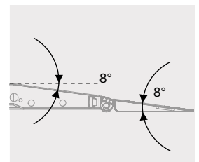
MFL 115 Bakparti med ramp, fällbar mot flakbotten för större plan flakyta. Passar ej på släp.
